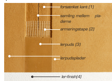
forsænket kant (1), armeringstape (2), lerpuds (3) and ler-finish (4)
